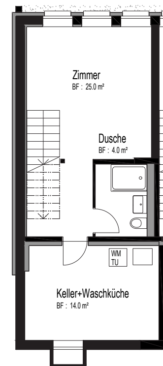
Untergeschoss
