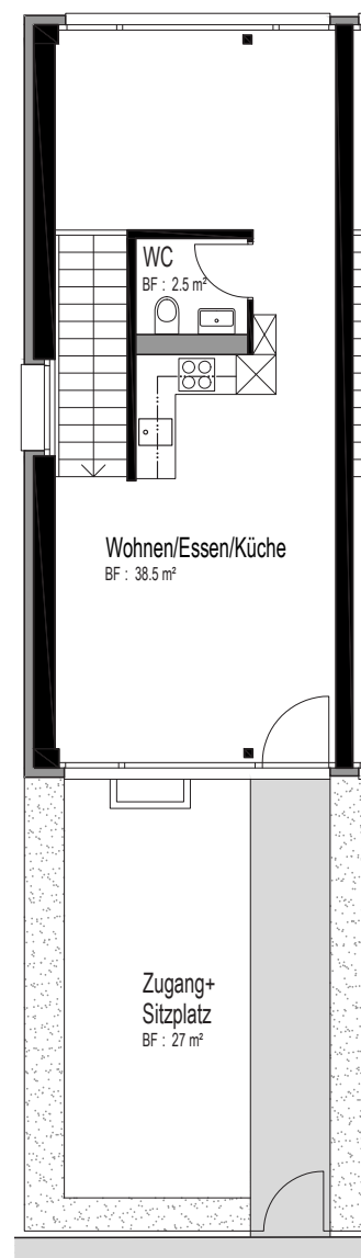
Erdgeschoss
